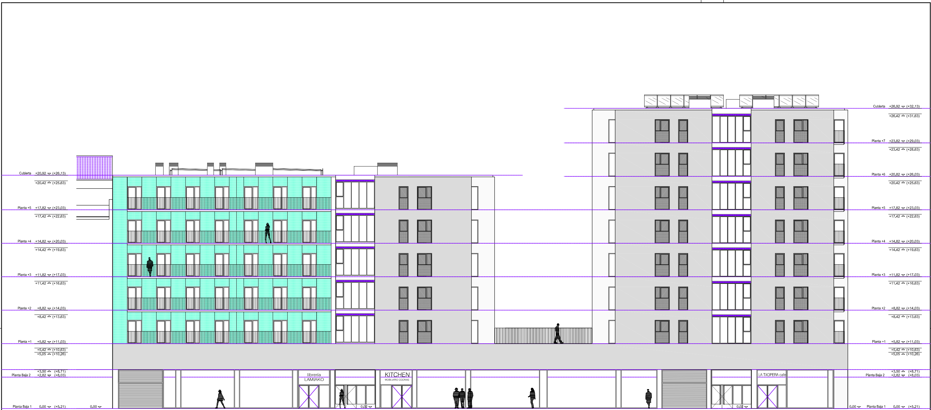
ALZADO A-B (SUR)
