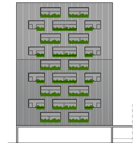
alzado sur e:1/500
