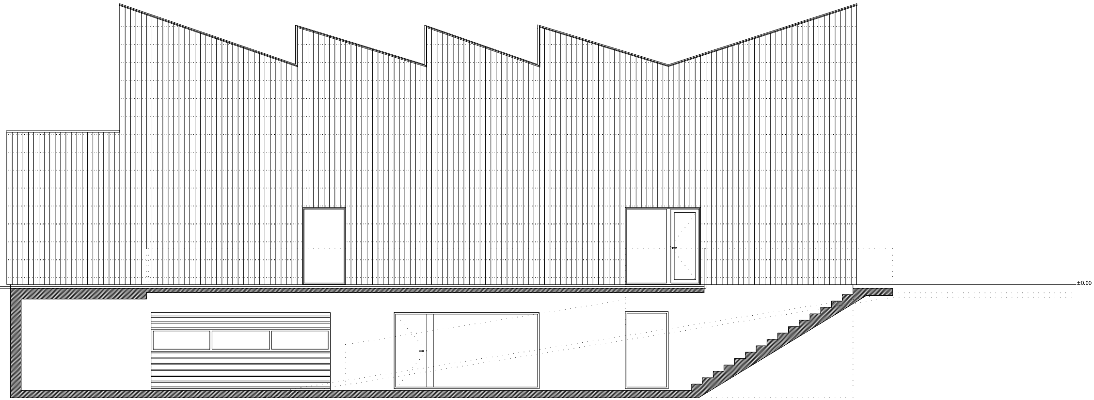
ALZADO CD
