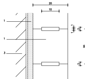
DETALLE F PLANTA E 1/5
