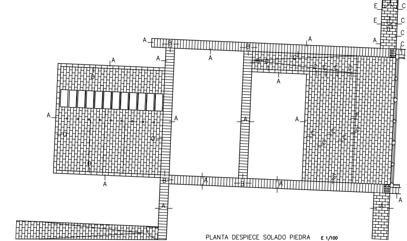
PLANTA DESPIECE SOLADO PIEDRA E 1/100 LOCALIZACION DETALLES
