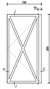
PUERTA P3 E 1/25 ALZADO INTERIOR
