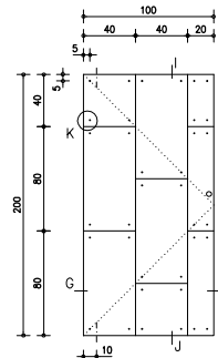
PUERTA P3 E 1/25 ALZADO EXTERIOR
