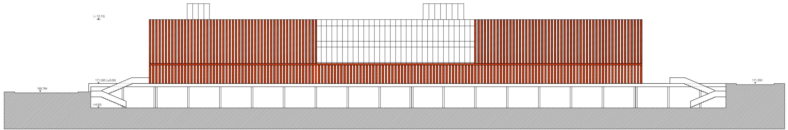
ALZADO A-B
