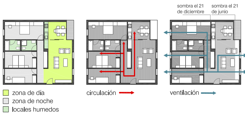
planta tipo 1/600
