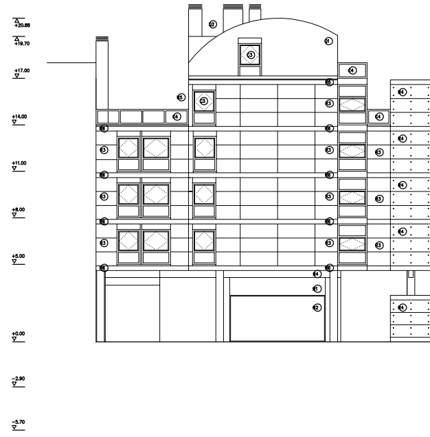
ALZADO CALLE FUEROS
